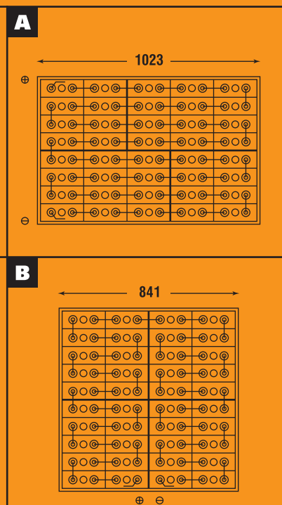
DIN 43536 - 80 Volts
