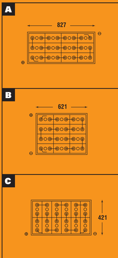
DIN 43535 - 24 Volts
