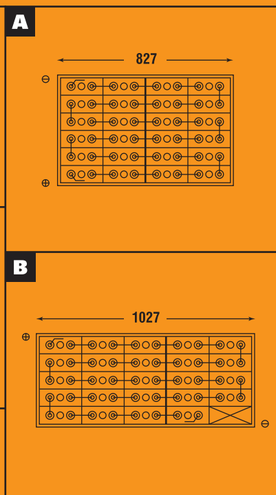
DIN 43531 - 48 Volts
